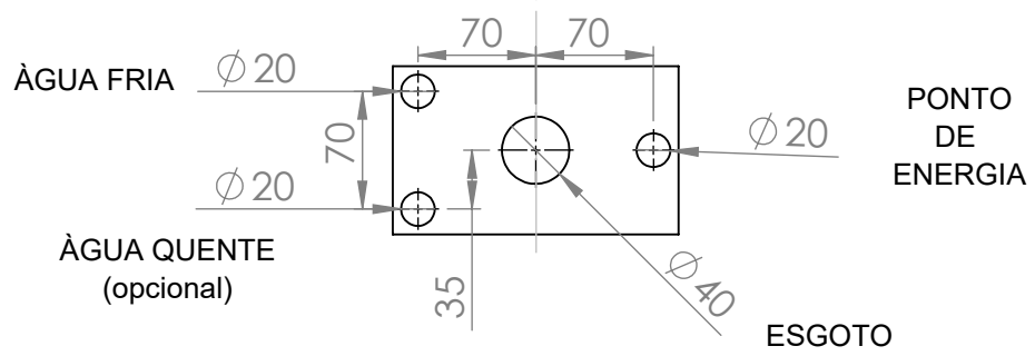
Esquema de instalação (Sob acento)
